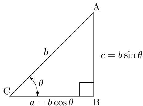
図 11 三角関数
