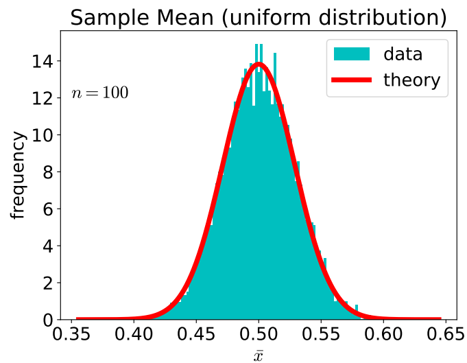
図 2 [0, 1) の一様分布に対する標本平均の分布。標本サイズは 100
